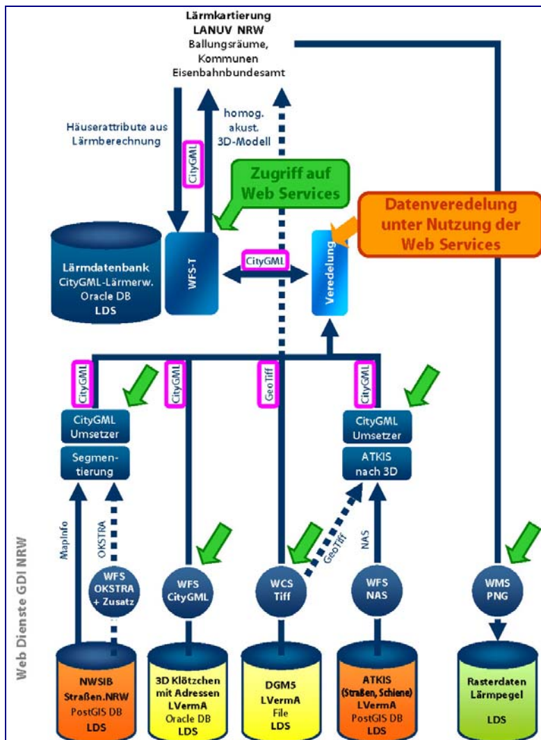
Abb. 2: Web Service-Architektur der Umsetzung der EU-Umgebungslärmkartierung in NRW (Quelle: IGG Uni Bonn).
